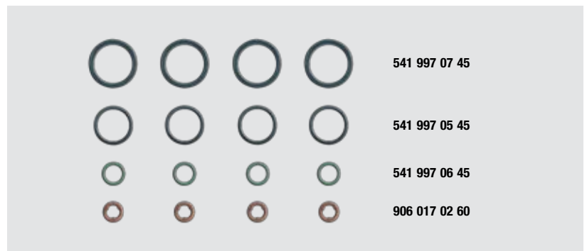
Bild1_OM 904 / OM 924, EinspritzdüSENSATZ 15-31357-02
